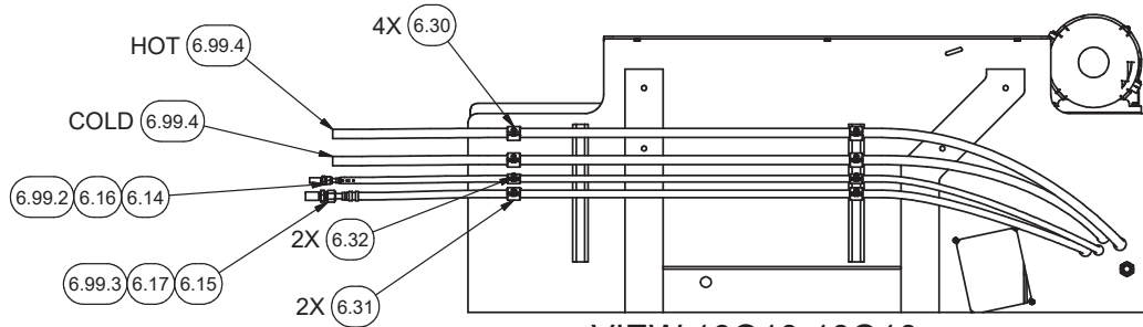
VIEW 10Q10-10Q10
