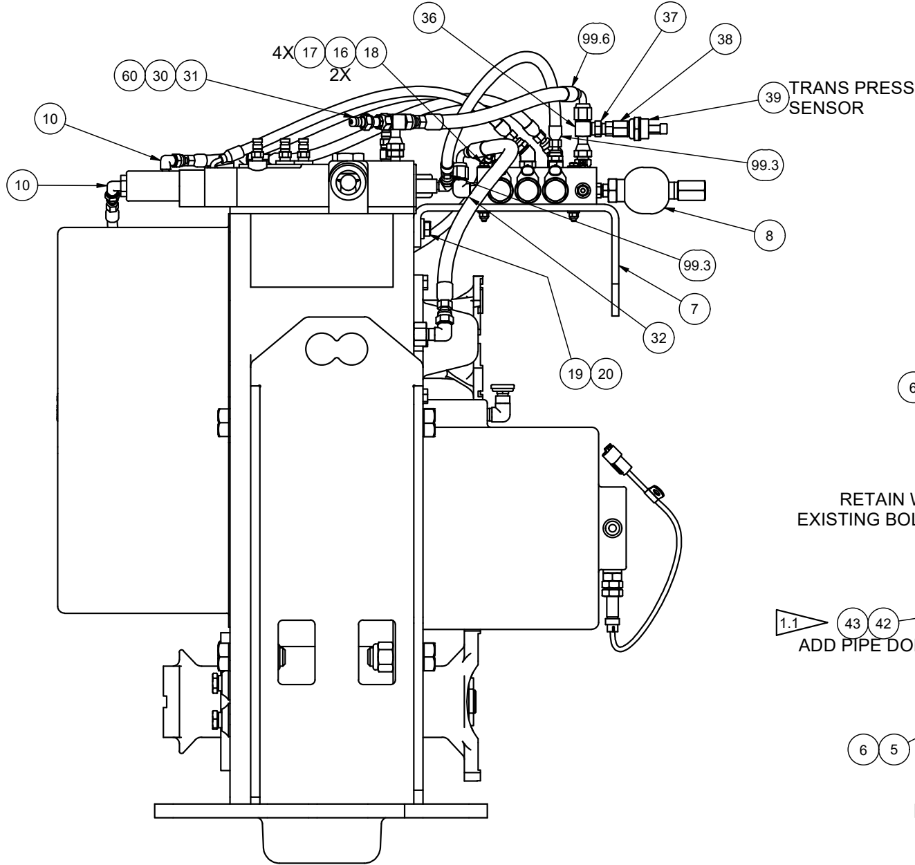
LEFT SIDE
