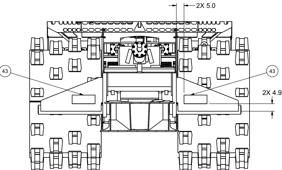
SECTION 4H2-4H2
