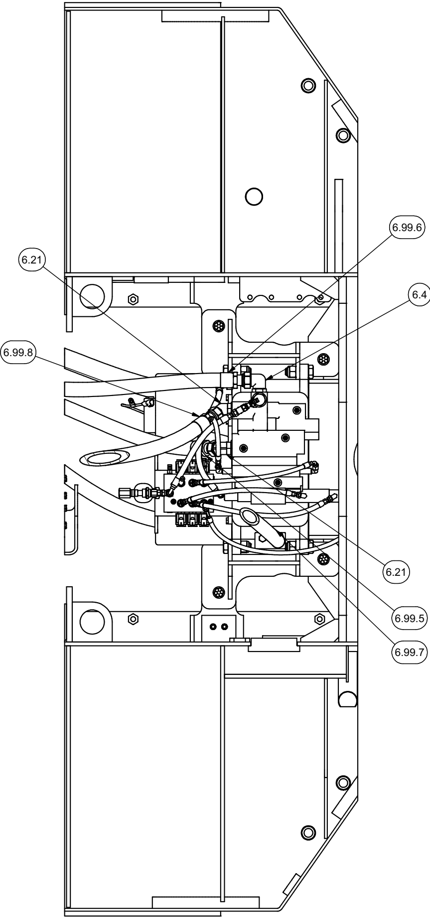
SECTION 12AC10-12AC10
