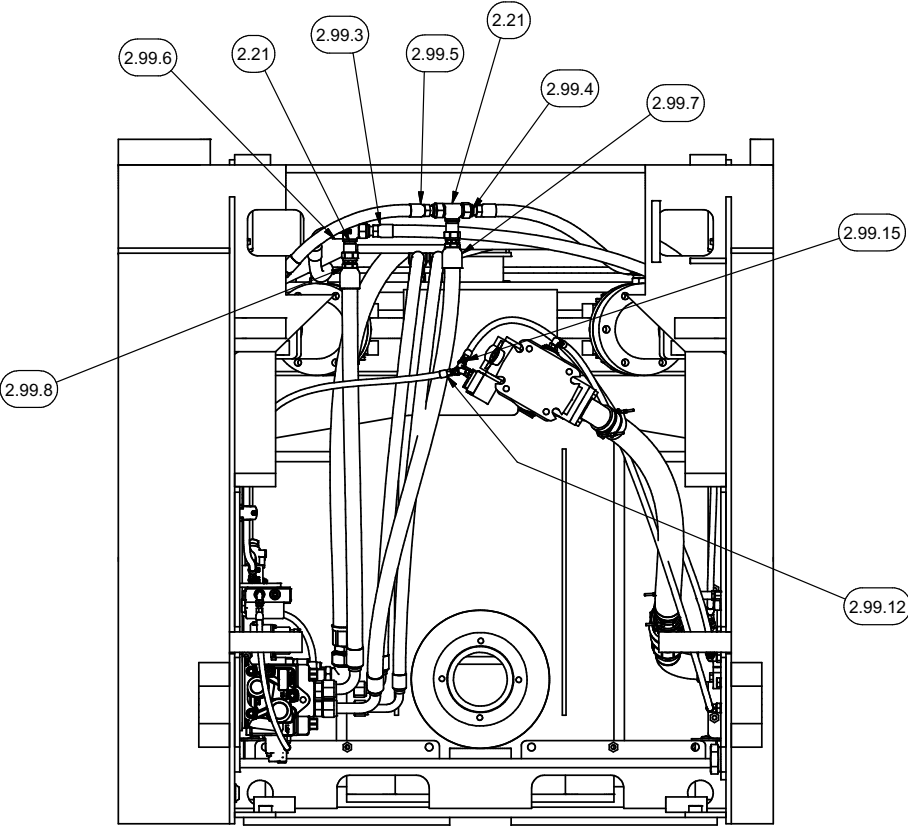
SECTION 4E3-4E3
