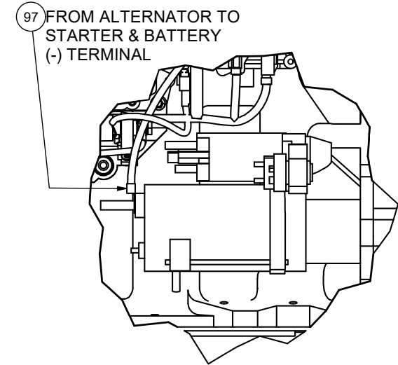
DETAIL 2B2 ALTERNATOR & STARTER (-) LUG
