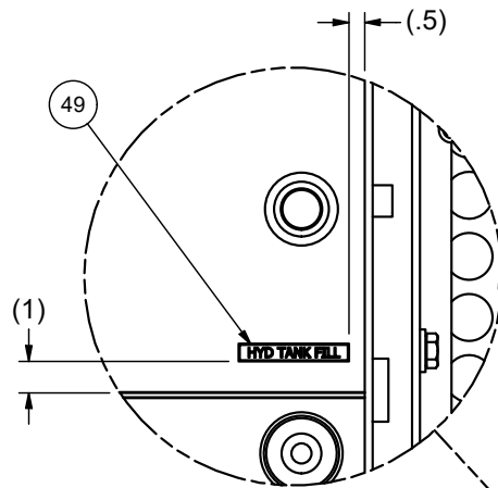
DETAIL 4G4 HYD TANK FILL
