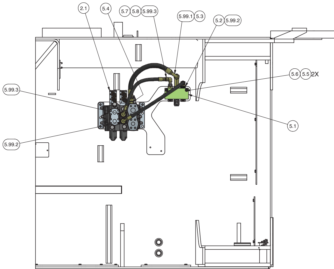
SECTION 9AB9-9AB9
