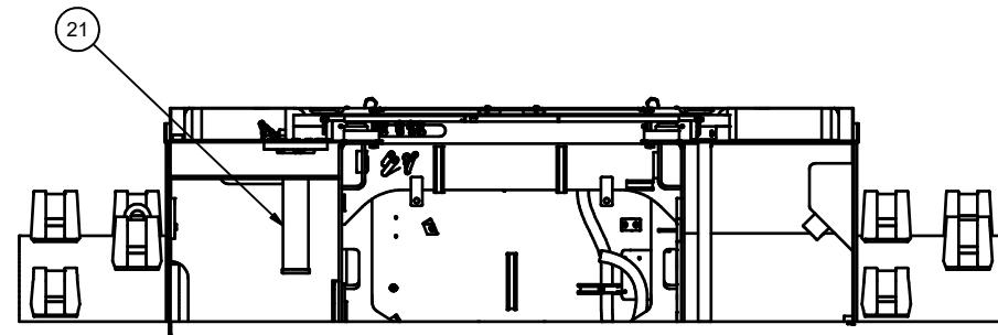
SECTION 3M2-3M2
