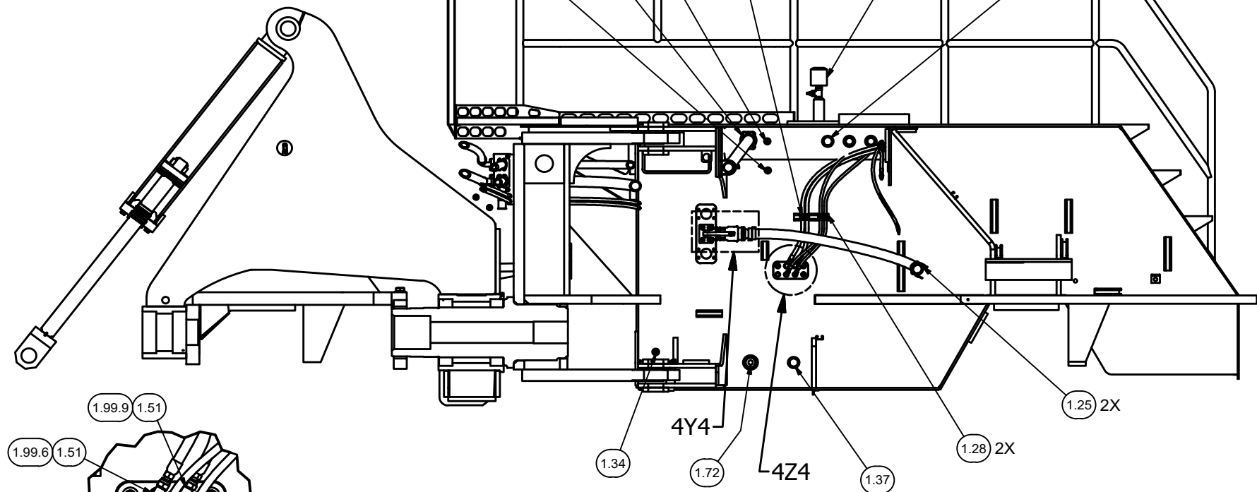
SECTION 4E2-4E2
