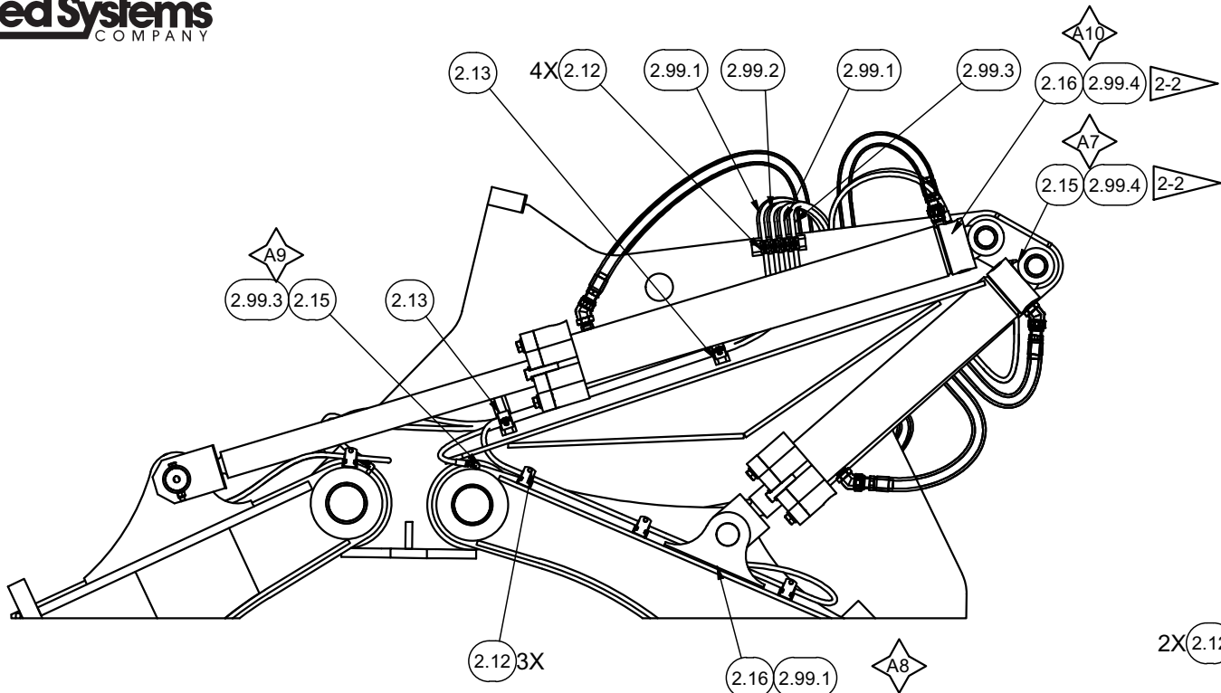
SECTION 3B2-3B2
