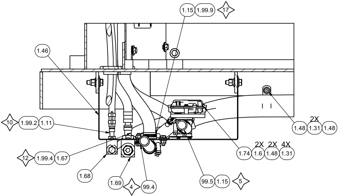
SECTION 4E4-4E4
