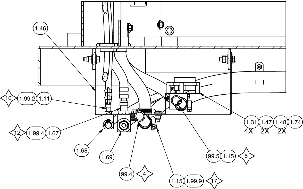
SECTION 3E3-3E3
