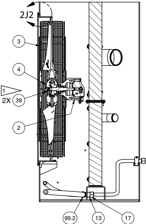
SECTION 2H1-2H1
