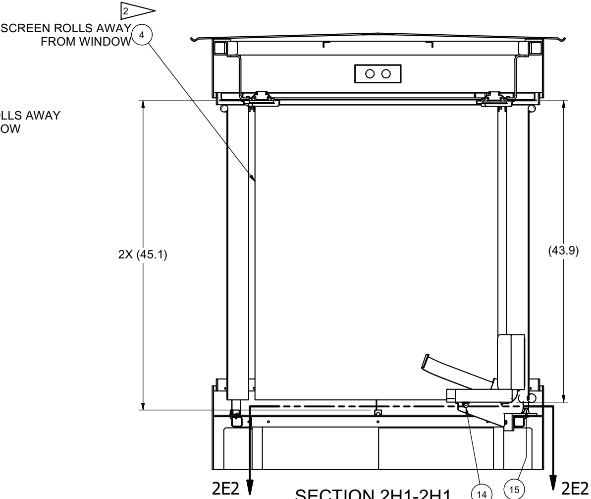
SECTION 2H1-2H1
