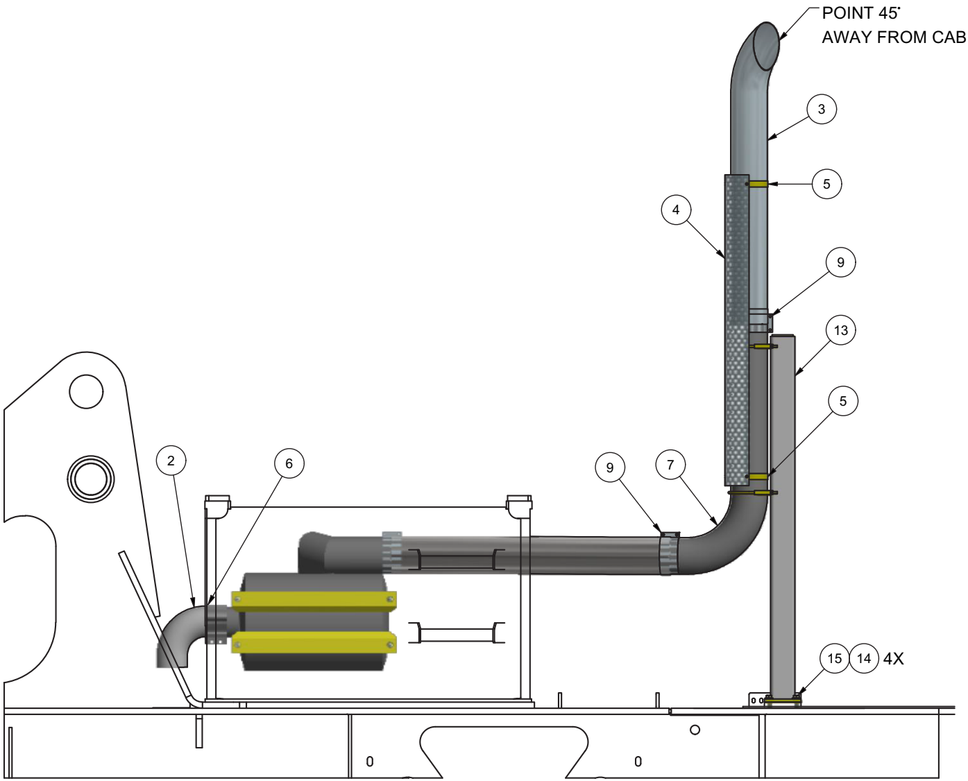
VIEW A-A
