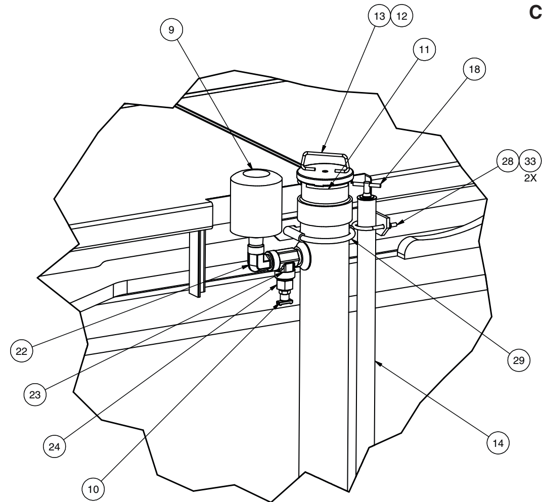
DETAIL 2E
