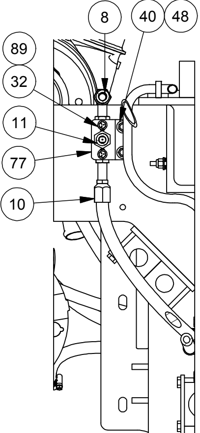
SECTION 4E-4E
