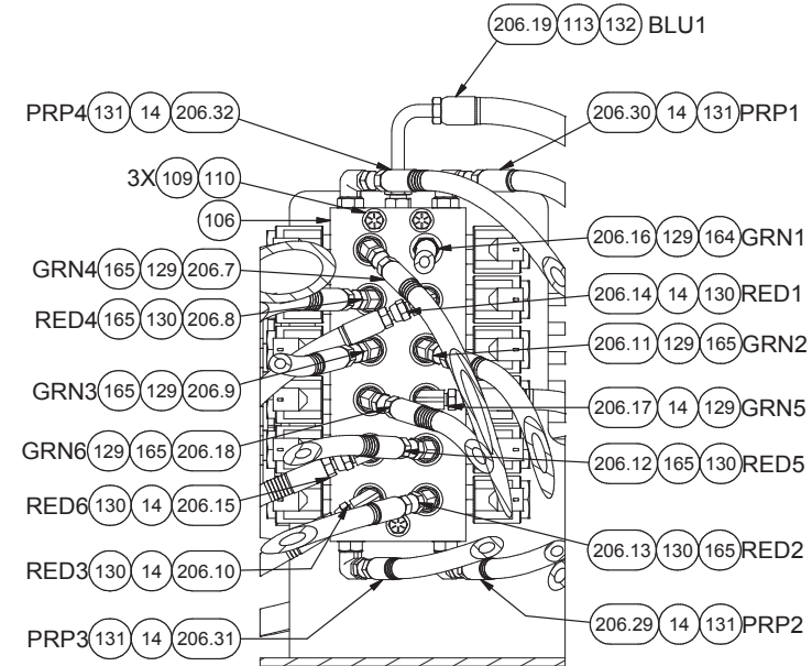
SECTION 3E-3E
