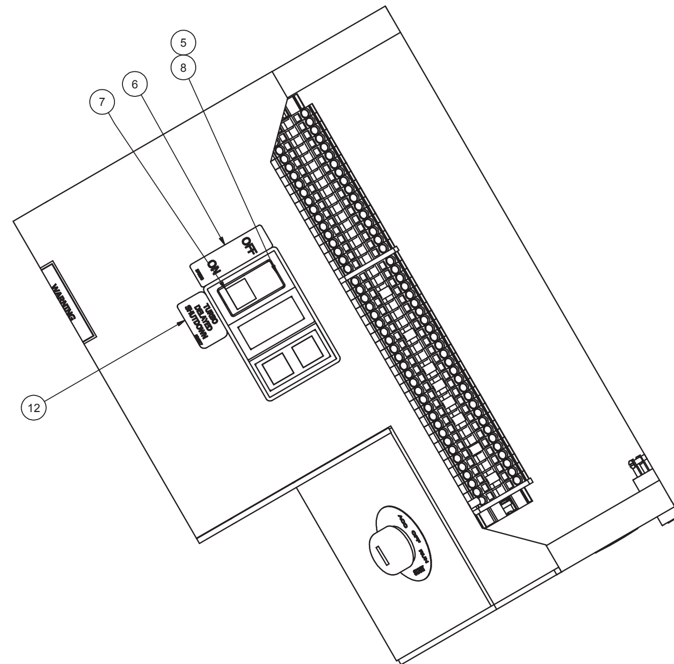
SECTION A-A
