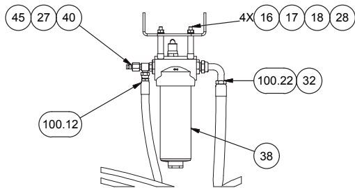
SECTION 3H-3H
