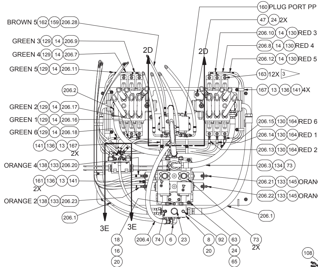
SECTION 2B-2B
