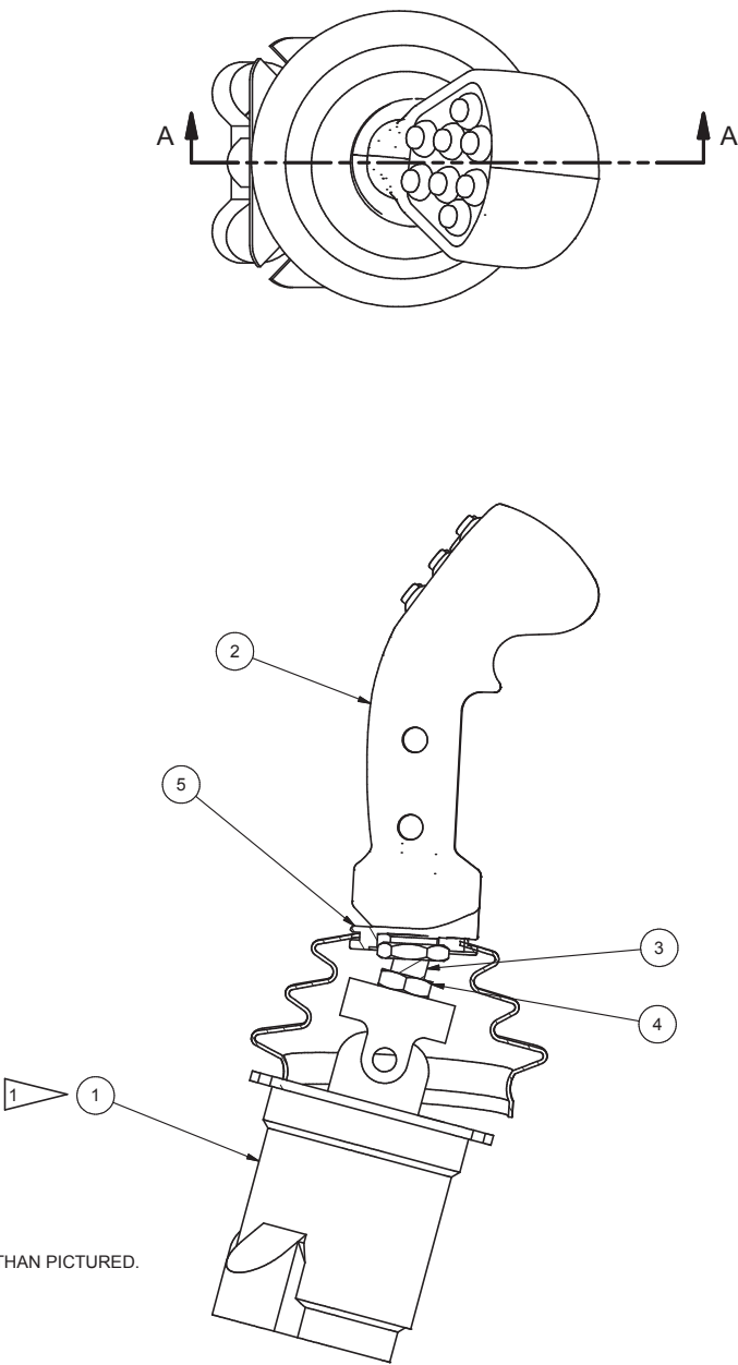
SECTION A-A
