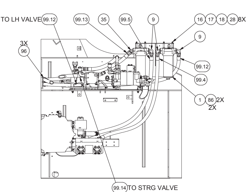
SECTION 2A-2A
