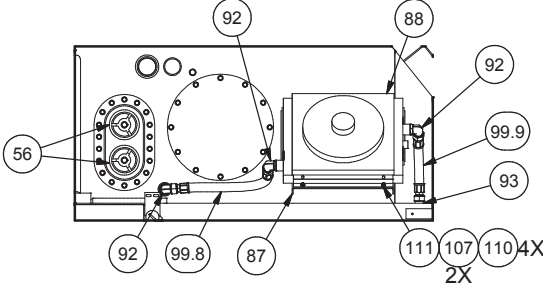
DETAIL 2E
