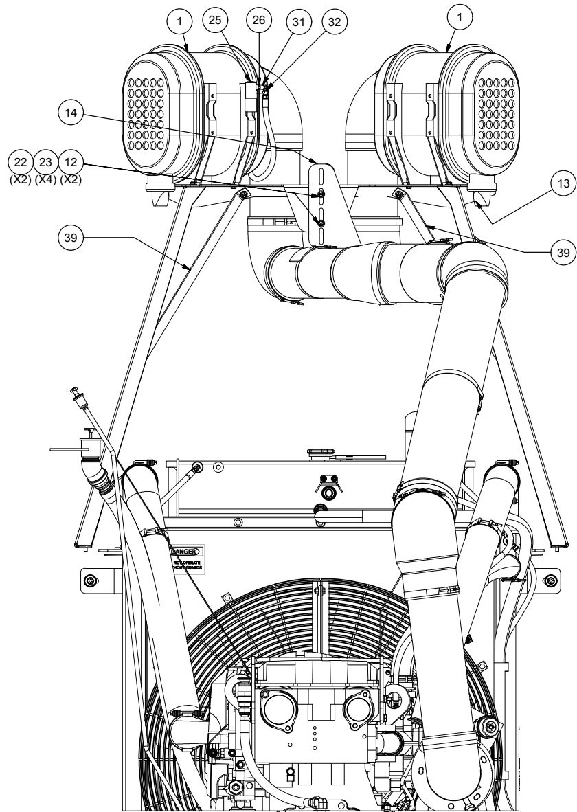
SECTION 2A-2A
