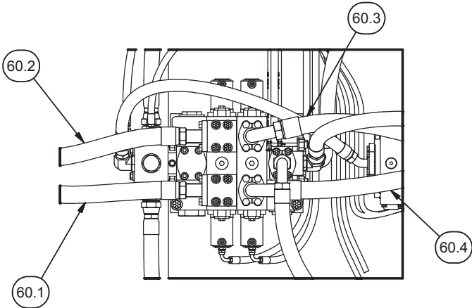
DETAIL 4E
