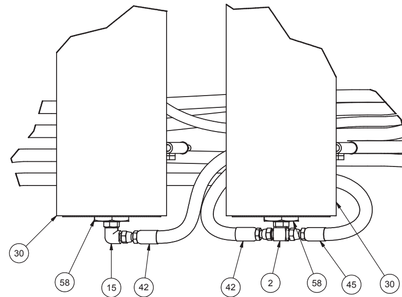
DETAIL 3E
