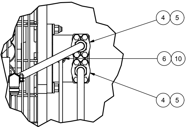
DETAIL 3E
