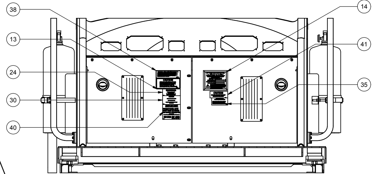
SECTION 4E-4E
