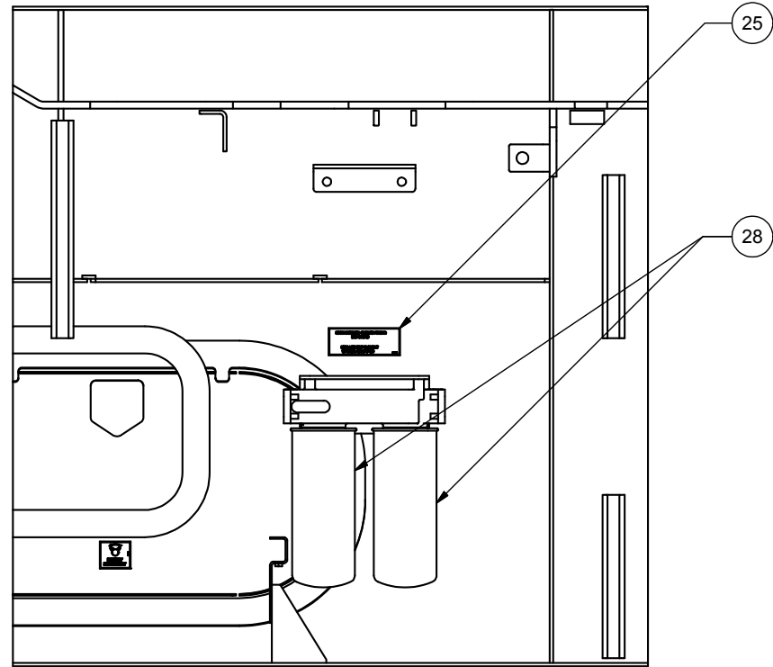
SECTION 3H-3H
