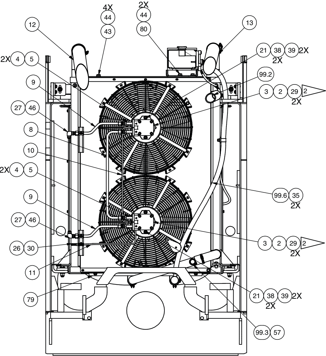
SECTION 2B-2B
