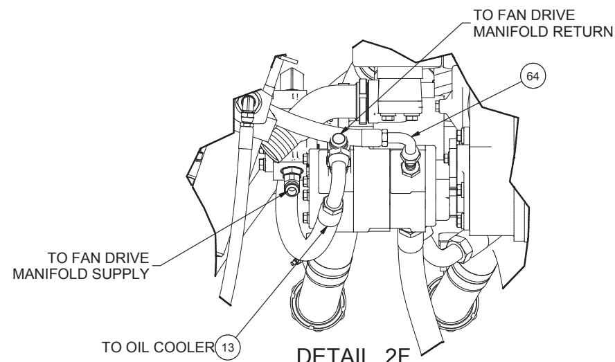
LEFT SIDE
