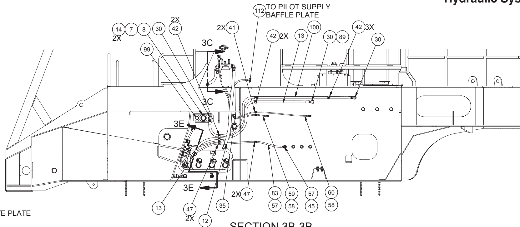
SECTION 3B-3B
