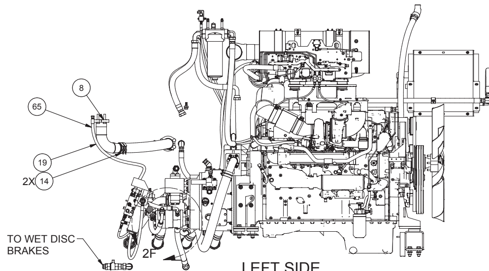
LEFT SIDE
