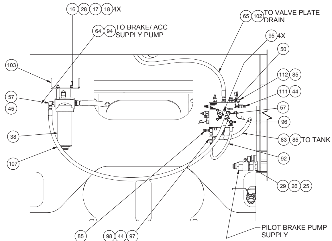
SECTION 3E-3E
