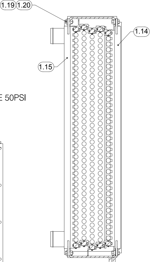
SECTION A-A
