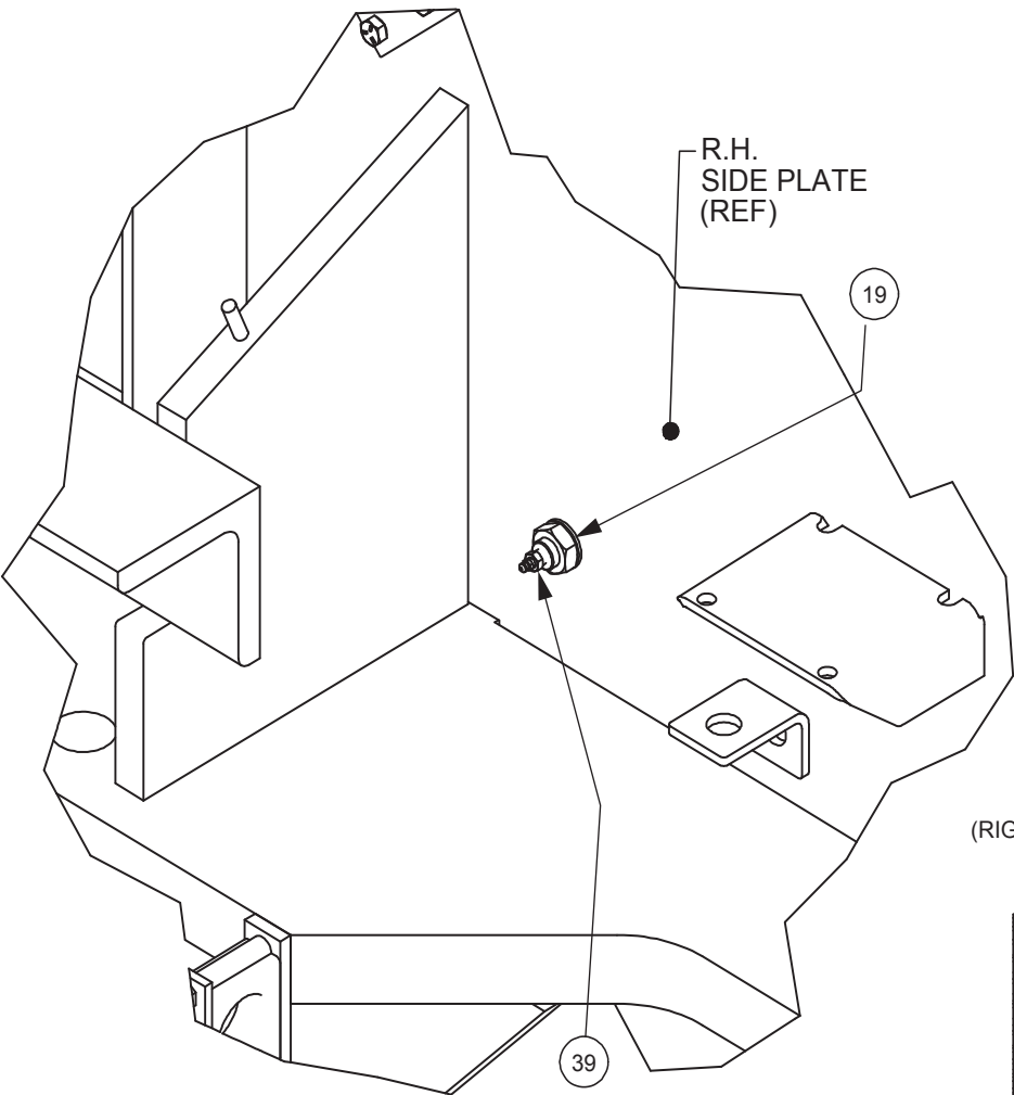
BRAKE BLEEDER INST (TYP)
