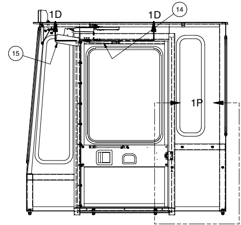
SECTION 1B-1B
