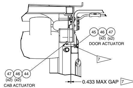
DETAIL 1E DOOR SWITCH INSTALLATION
