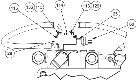
DETAIL 3E
