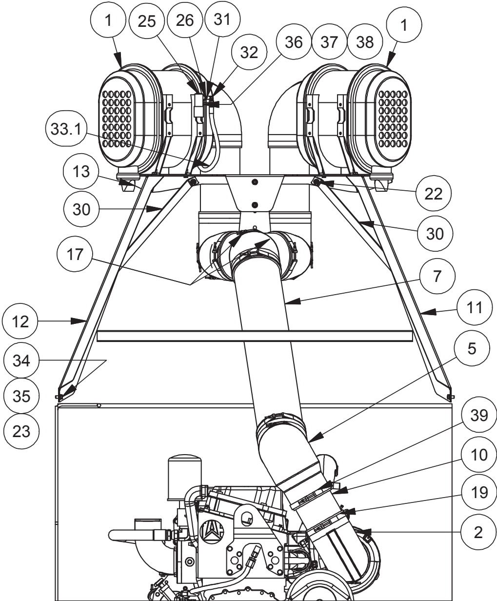
SECTION A-A
