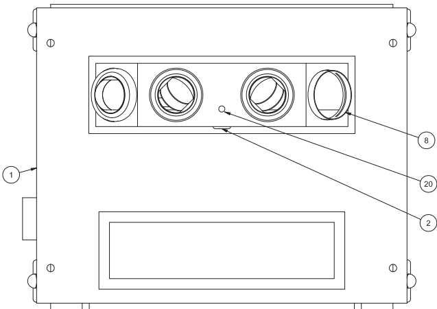
VIEW A-A
