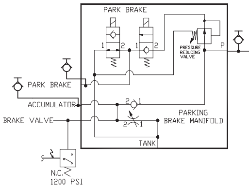
ANSI SCHEMATIC
