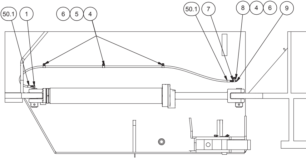
SECTION 1E2-1E2
