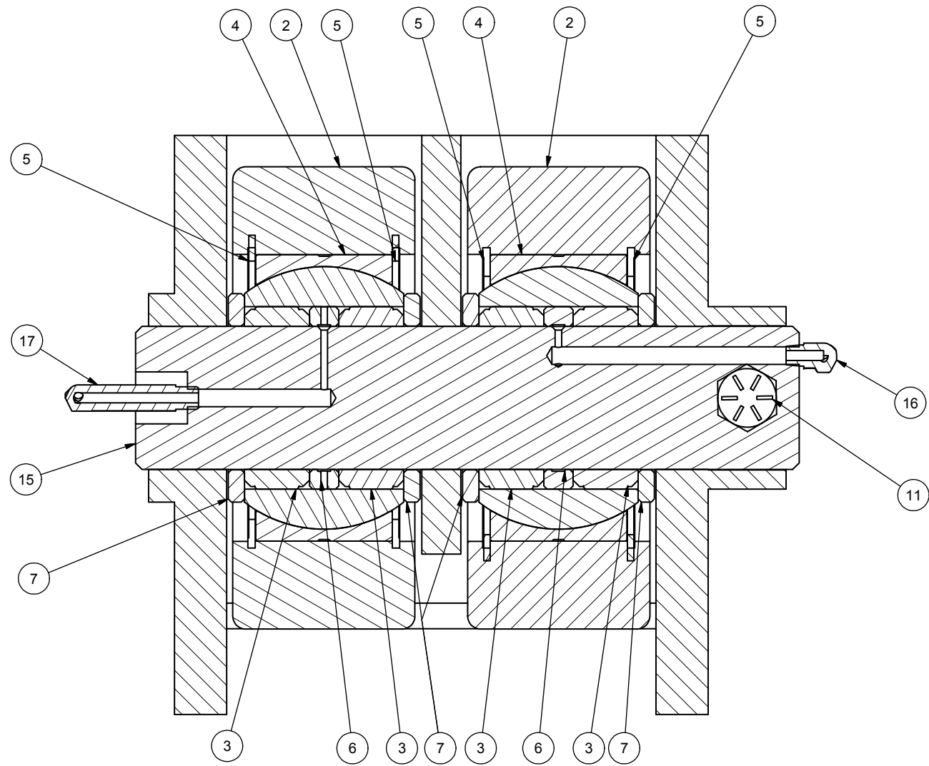
SECTION A-A
