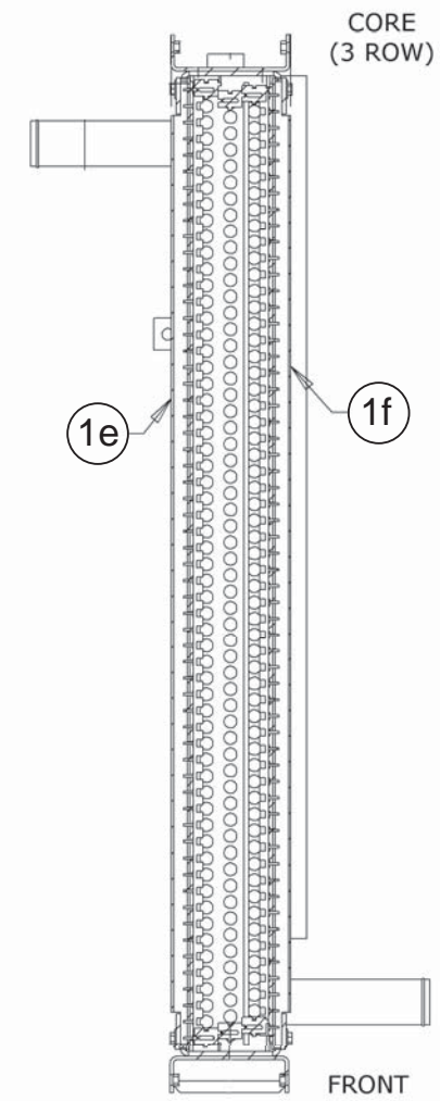
SECTION A-A
