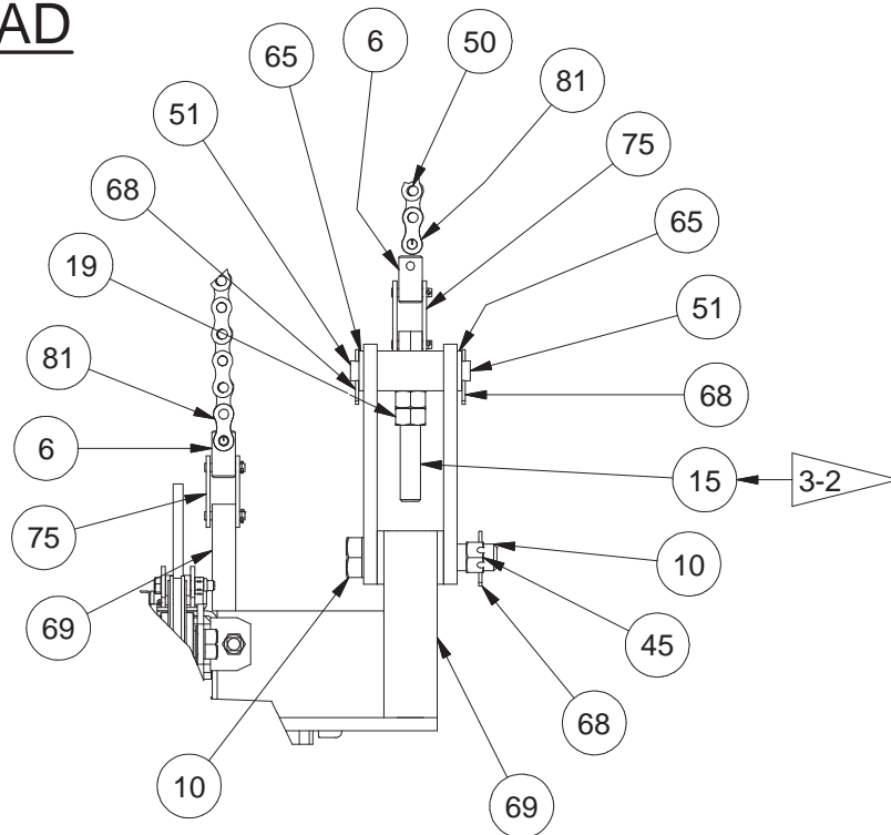
DETAIL AF
