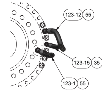
SECTION M3-M3 RH
