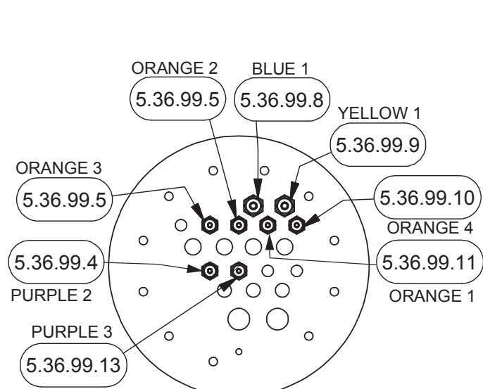
SECTION 10P-10P
