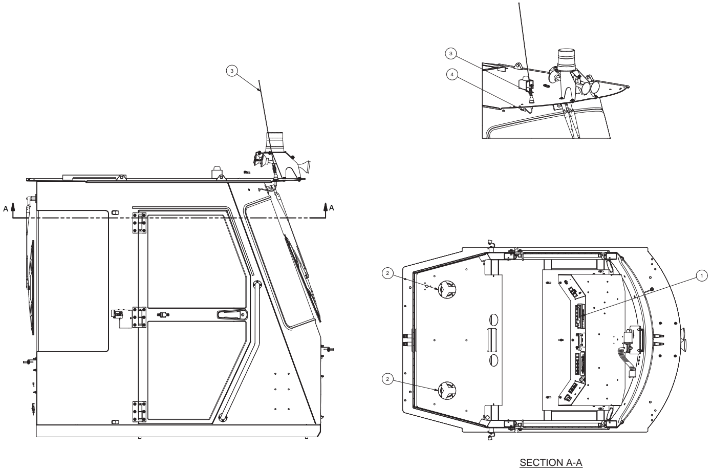
SECTION A-A
