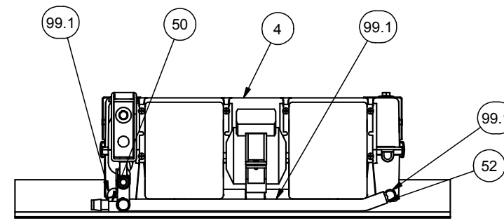
SECTION 3H-3H
