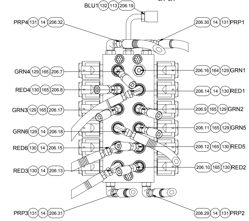
SECTION 2A-2A
