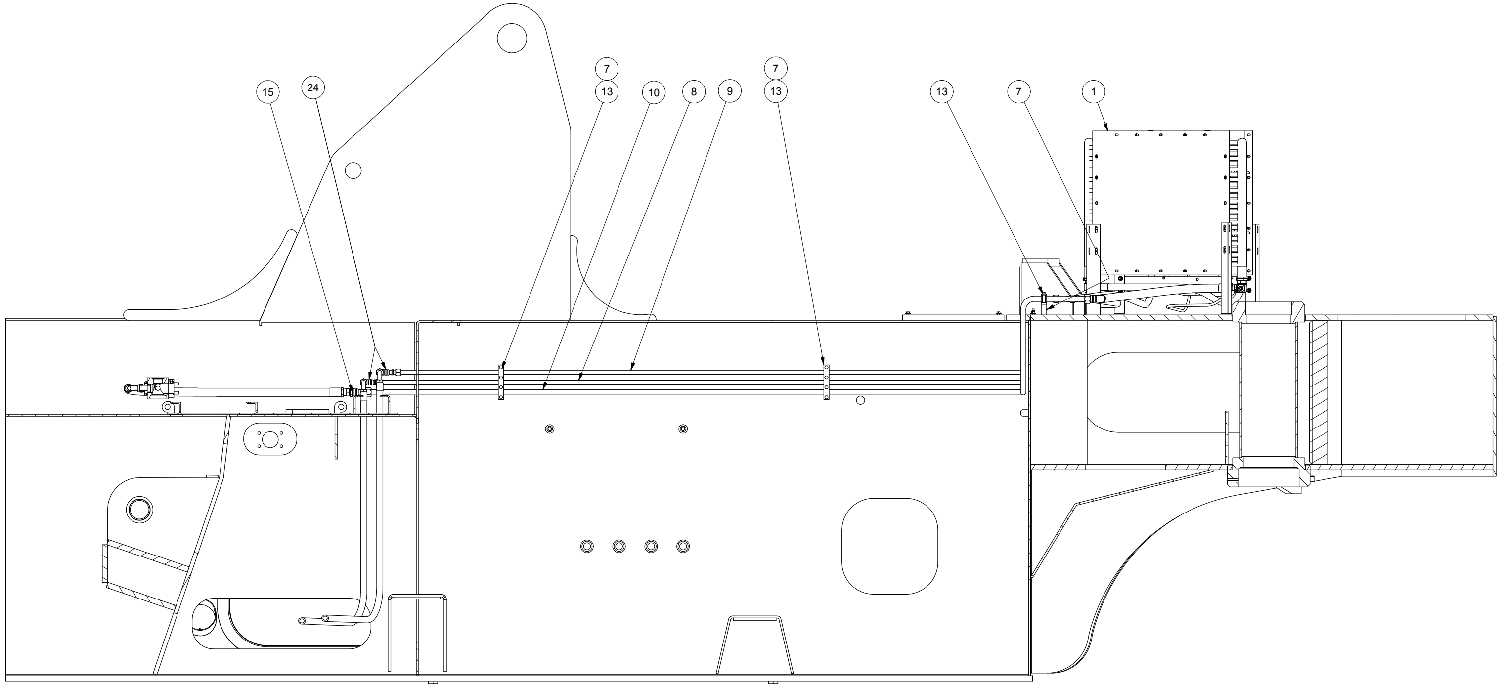
SECTION A-A
