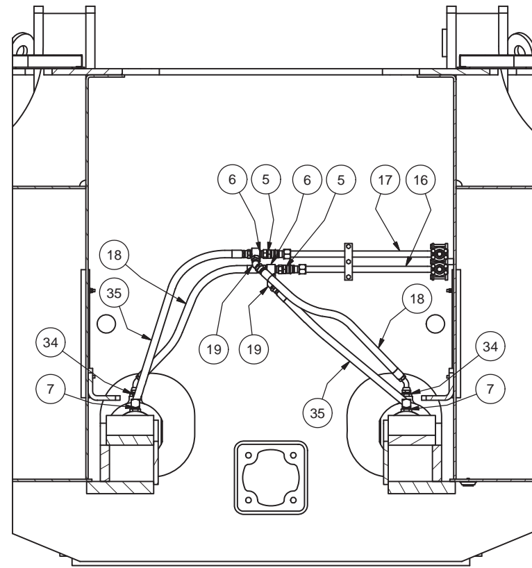
SECTION A-A
