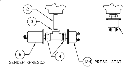
VIEW B-B SCALE: 1=8
